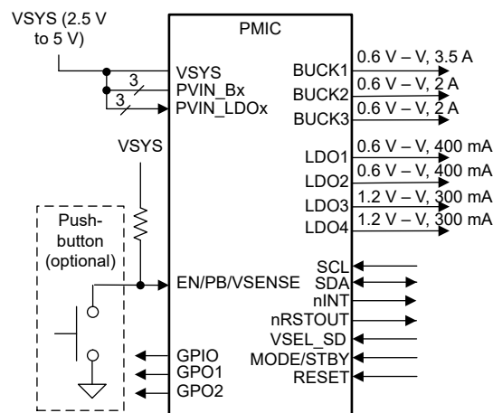
图 2-1. TPS65219-Q1 简化原理图
