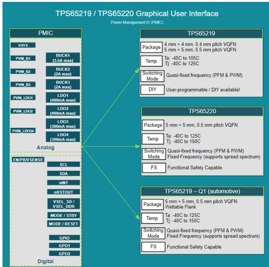
图 2-2. TPS65219-Q1 图形用户界面
