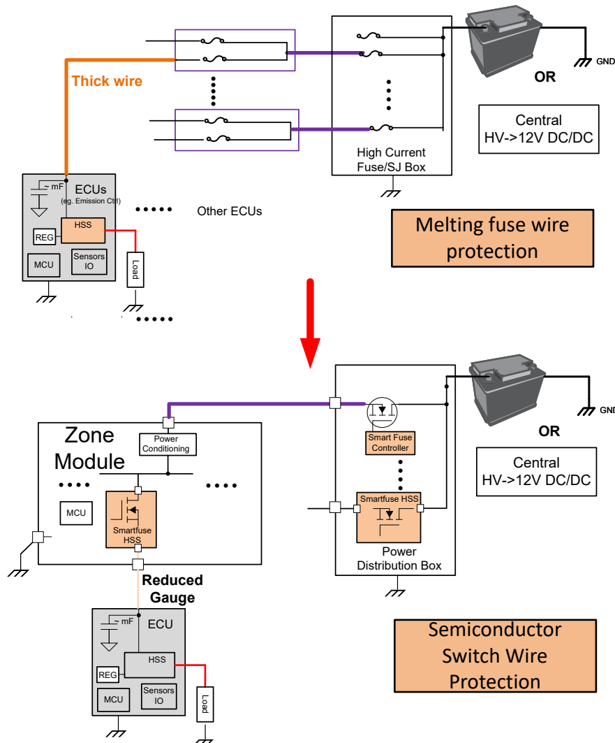
图 1. 区域控制器和配电盒中的熔断型保险丝替代产品
