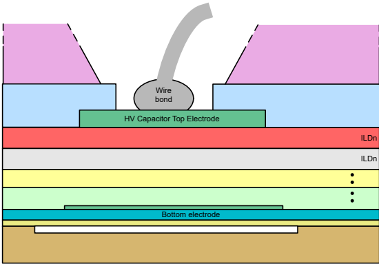
图 7. TI 高压隔离 SiO 2 电容器的横截面示例。
