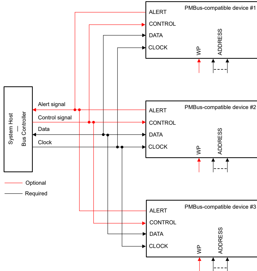
图 7-11. PMBus Connections
