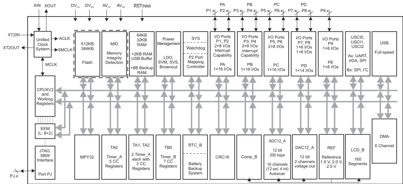
功能方框图 – MSP430F6659、MSP430F6658
