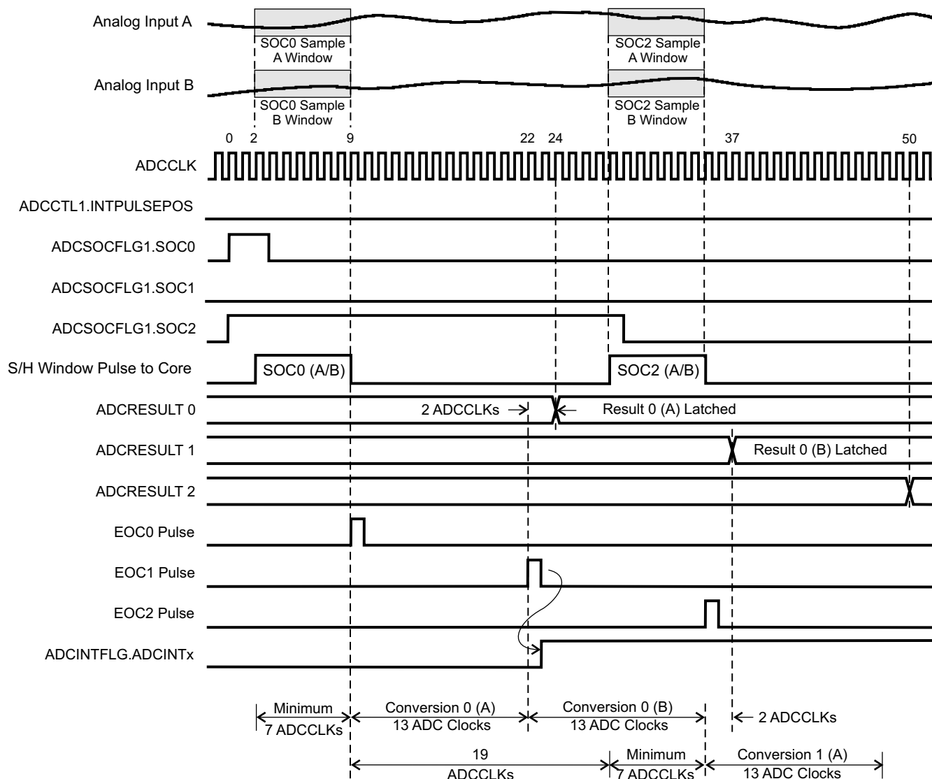
图 9-24. 同步模式/提前中断脉冲的时序示例
