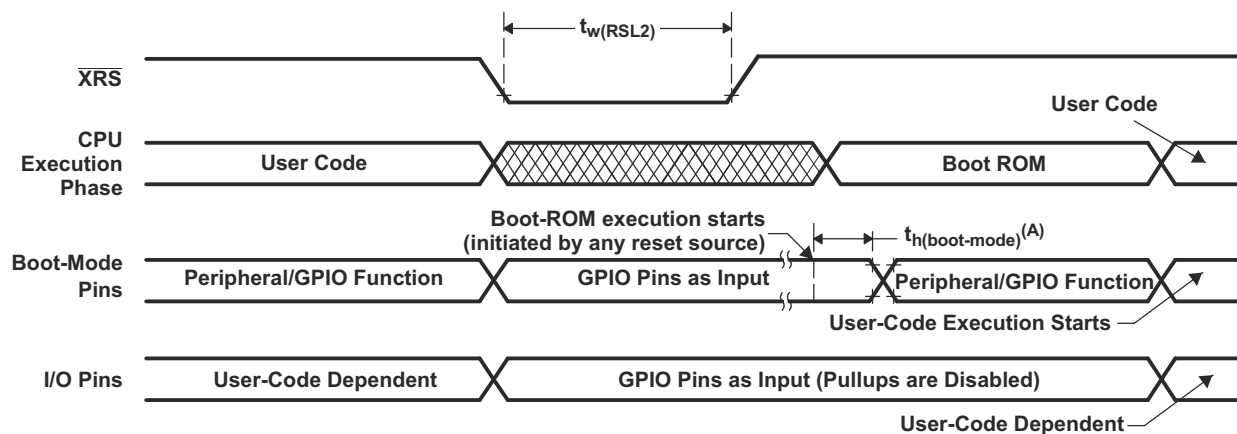
图 6-5. 上电复位
