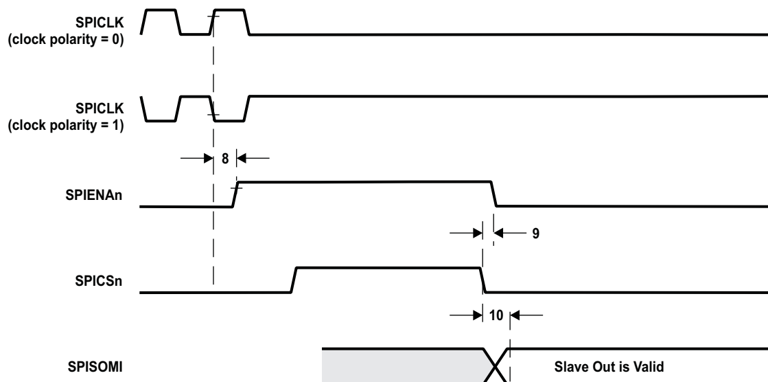
图 5-20. SPI 受控模式使能定时 (时钟相位 = 1)
