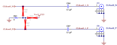
CLKout9
