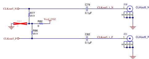
CLKout5
