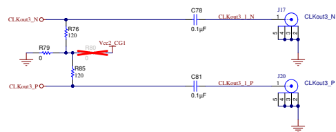
CLKout3
