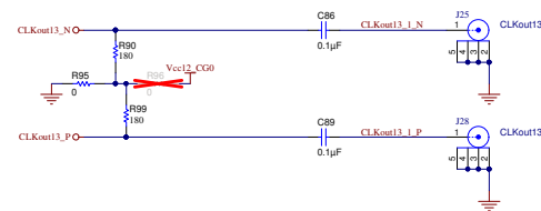
CLKout13
