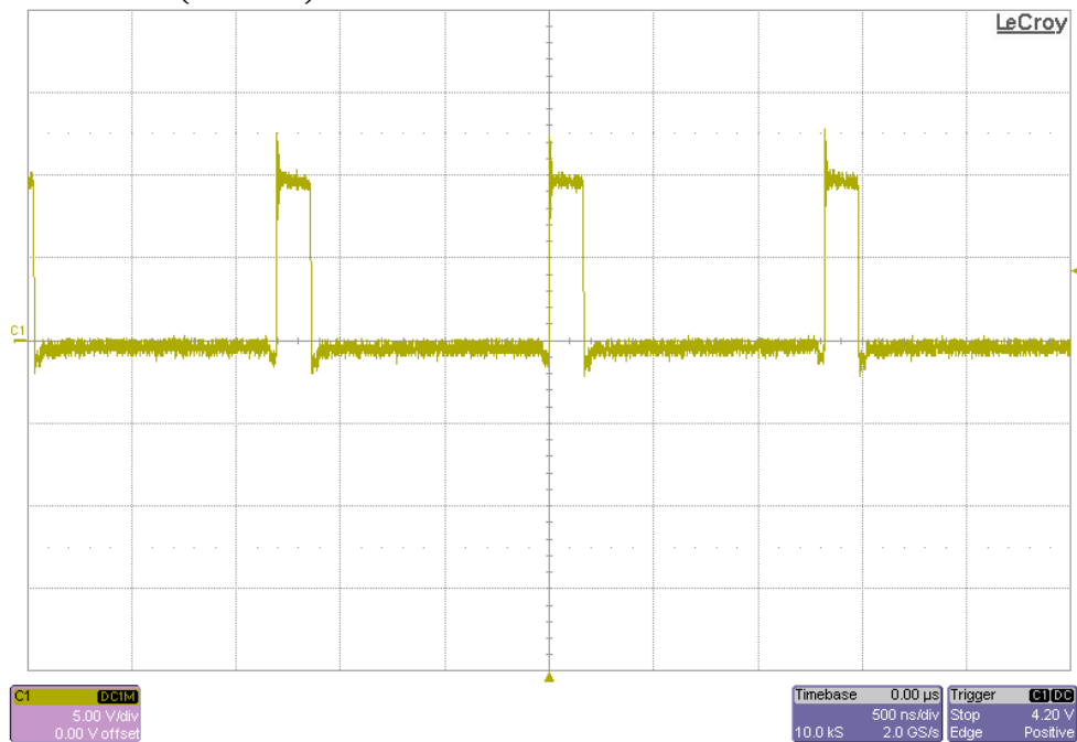
C1: VOUT_3A
