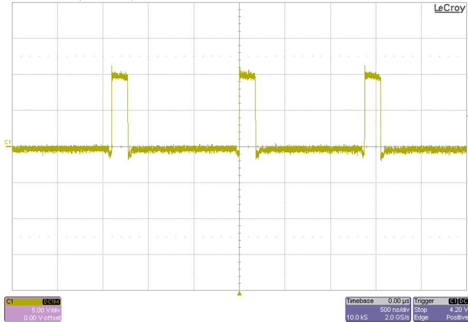
C1: VOUT_2A
