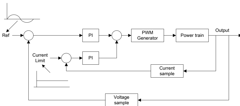
图 12. 逆变器环路控制框图
