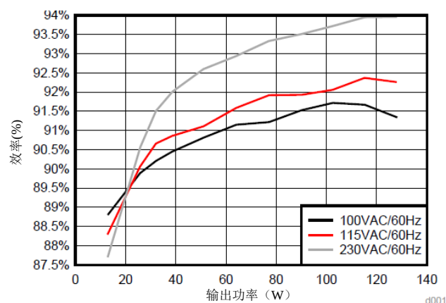
图 1.UCC28056 + UCC25630x 效率
