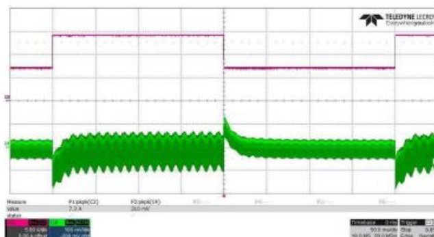
图 3.PMP21098 7A至14.2A瞬态响应
