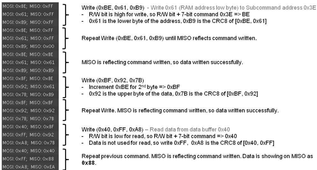
图 5-6. 读取启用保护功能 A
