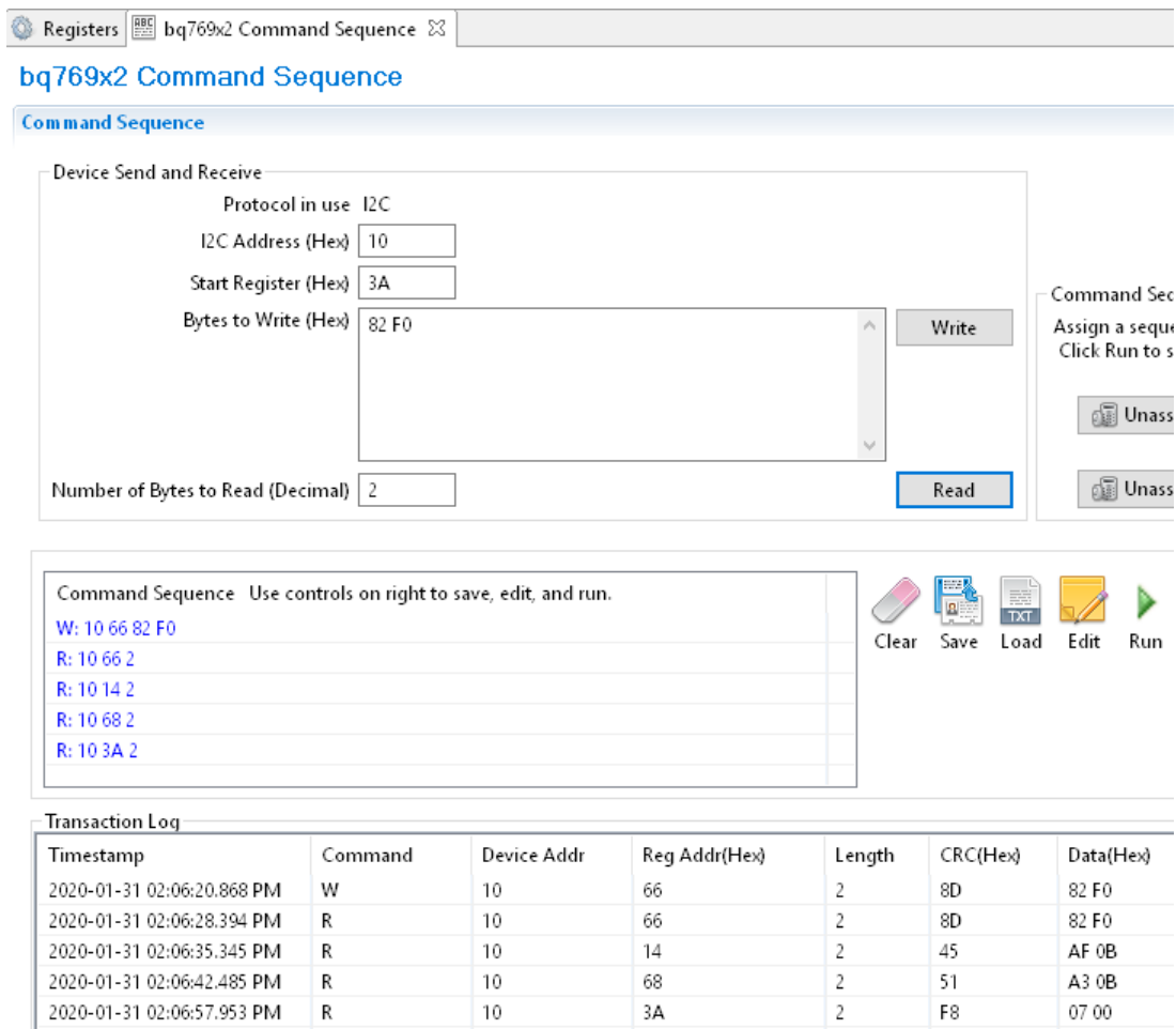
图 1-5. 显示执行多个直接命令的 BQStudio 示例
