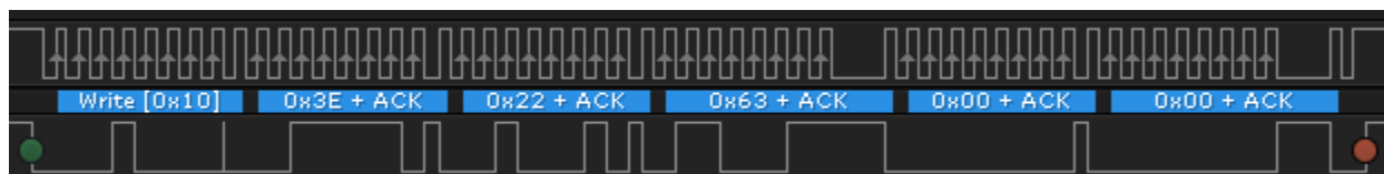
图 4-1. 使用 CRC 为 FET_ENABLE 子命令捕捉的 I2C 波形
