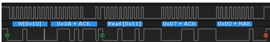
图 1-4. 为读取 CC2 电流捕捉的 I2C 波形
