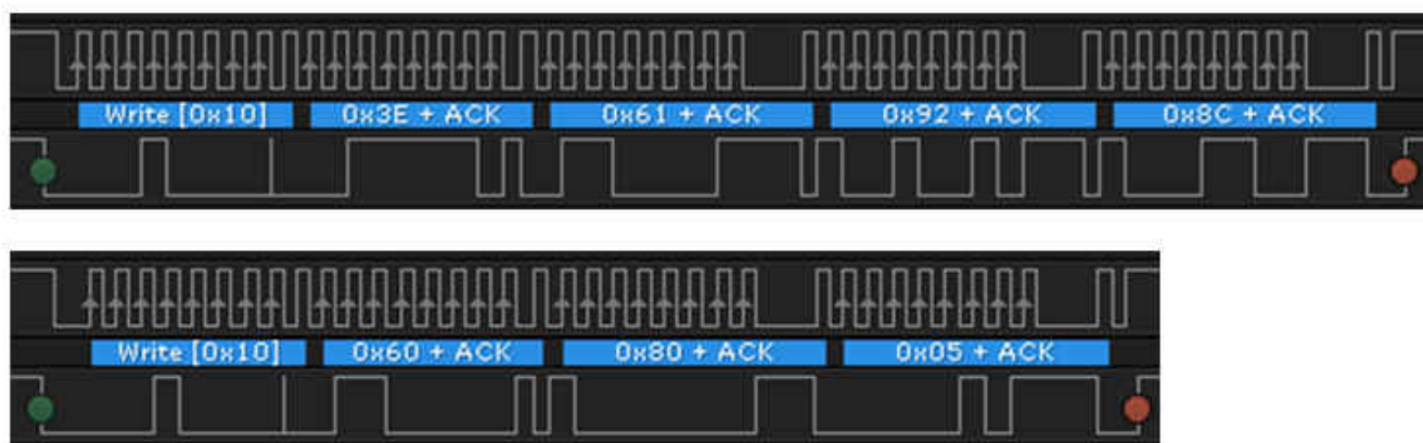
图 3-3. 为写入启用保护功能 A 捕捉的波形
