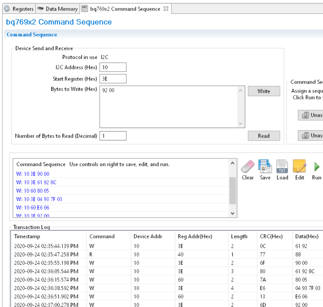
图 3-6. 显示执行 RAM 寄存器的读取和写入的 BQStudio 示例
