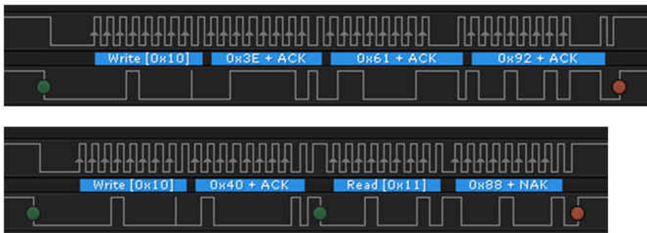
图 3-1. 为读取启用保护功能 A 寄存器捕捉的 I2C 波形
