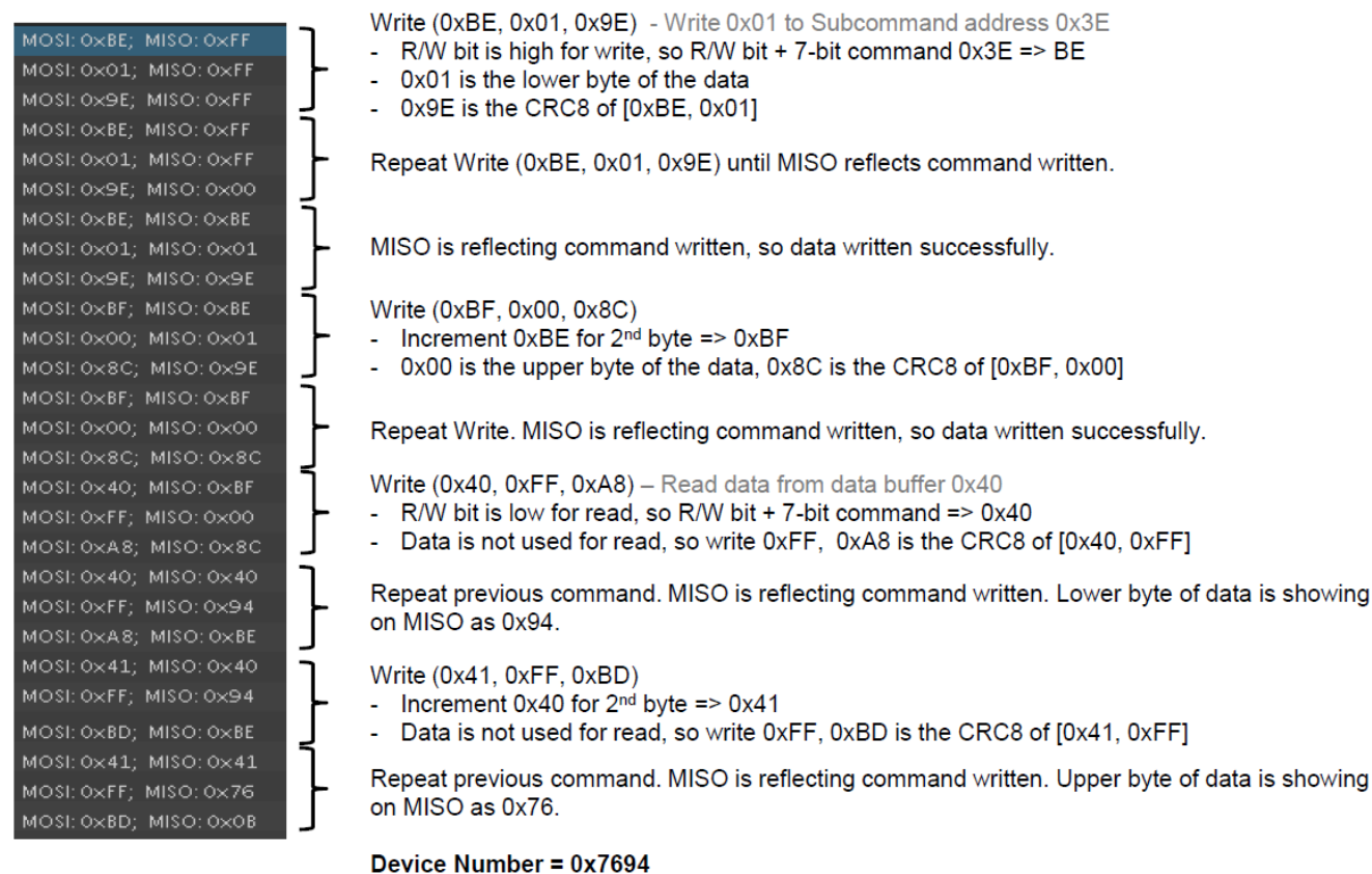
图 5-3. 器件型号子命令
