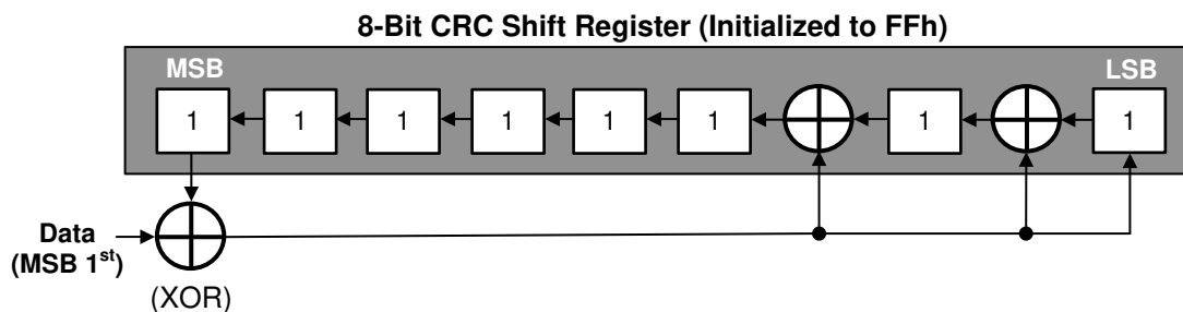
图 3-4. CRC-8-ATM (HEC) 硬件实现
