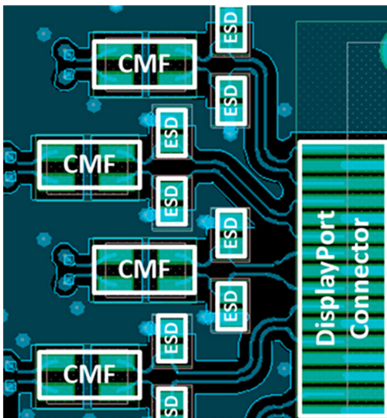
图 3-5. DisplayPort 放置
