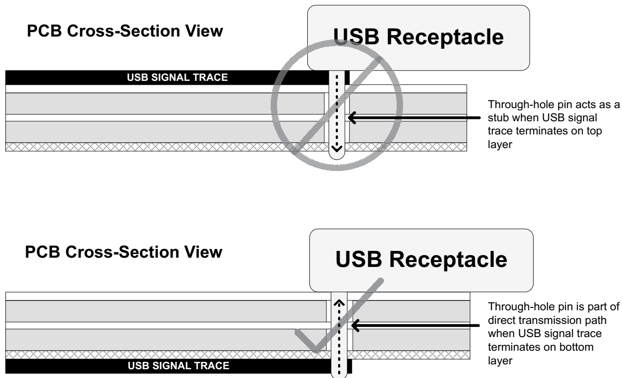
图 2-10. USB 穿孔插座连接
