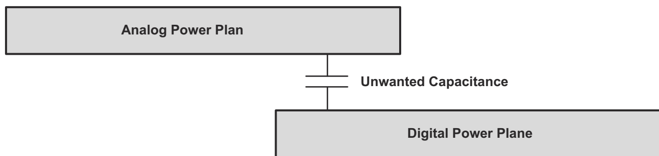
图 2-6. 重叠平面
