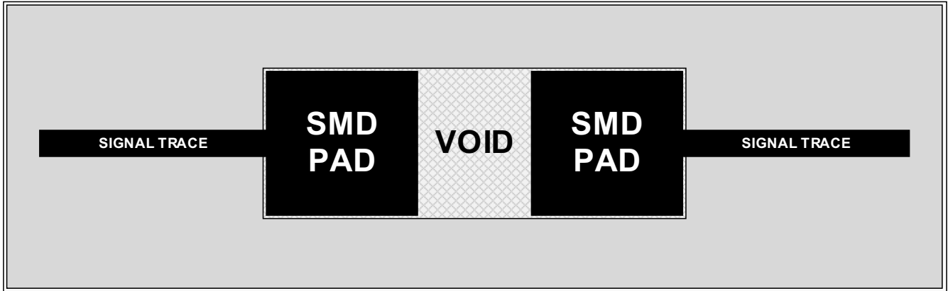
图 2-15. 表面贴装器件的参考平面空洞
