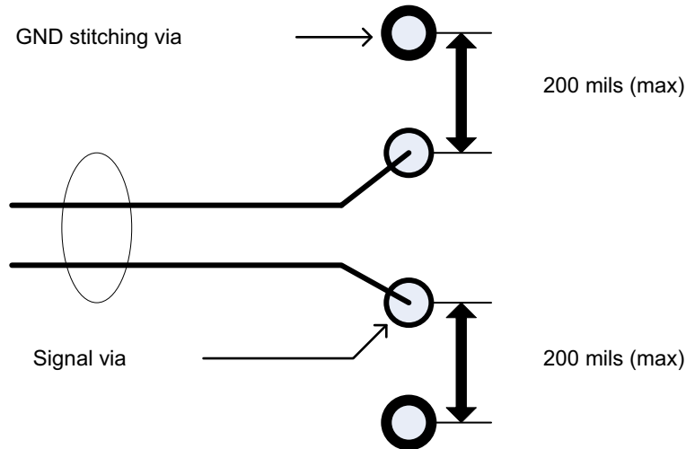
图 2-7. 拼接过孔
