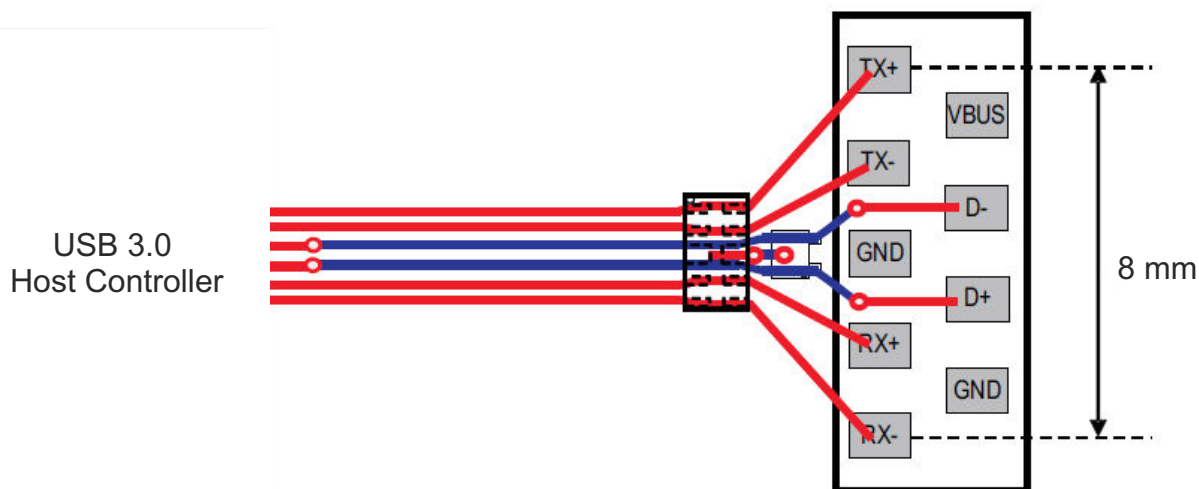
图 2-17. 直通布线
