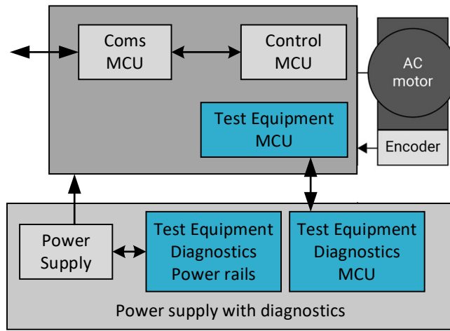
图3：架构3，具有单个安全MCU和PMIC（HFT=0，SIL 2）
