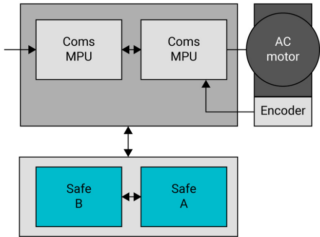
图 1：架构 1，具有双安全 MCU（HFT=1，SIL 2 或 SIL 3）
