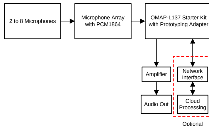
图 2. Block Diagram
