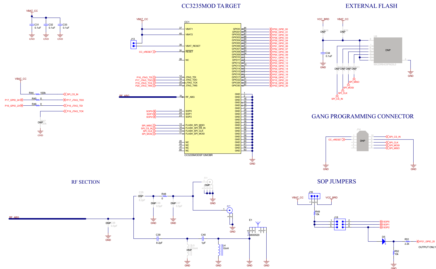
图 7-4. 原理图 (3/5)
