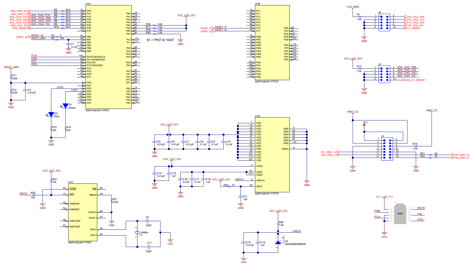
图 7-2. 原理图 (1/5)
