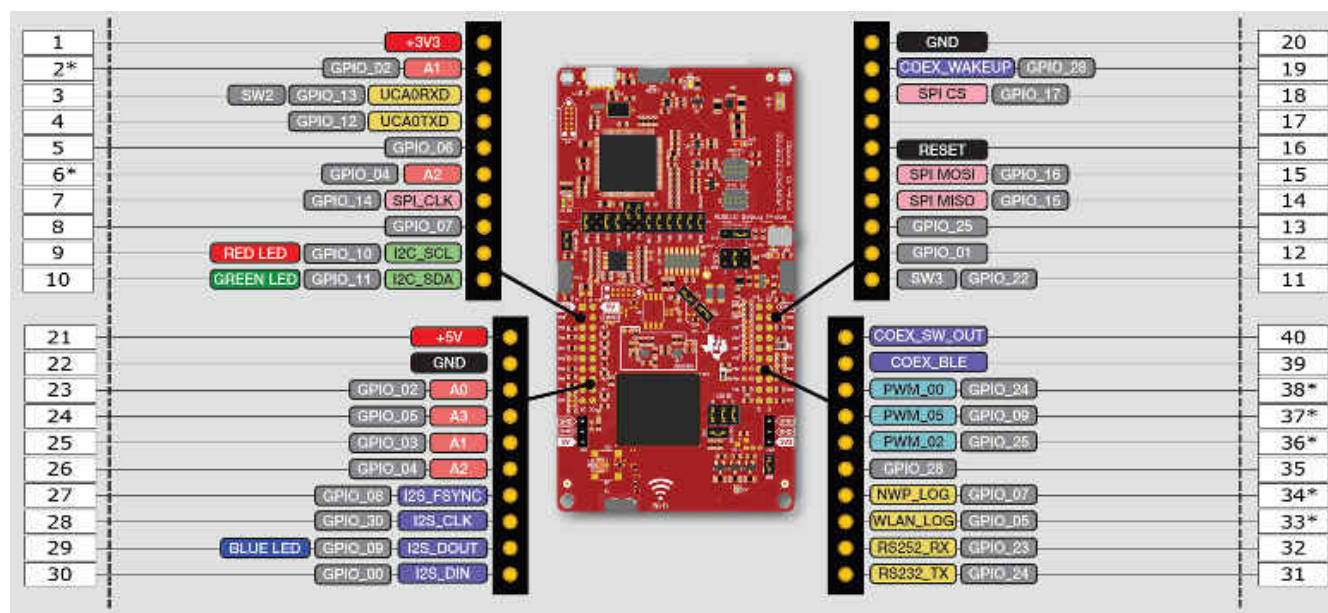
图 2-15. LAUNCHCC3235MOD BoosterPack 接头引脚分配
