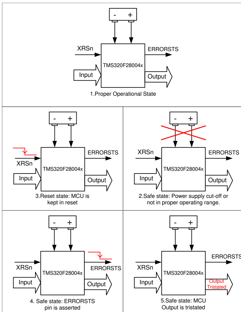
图 4-8. TMS320F28004x MCU 安全状态定义
