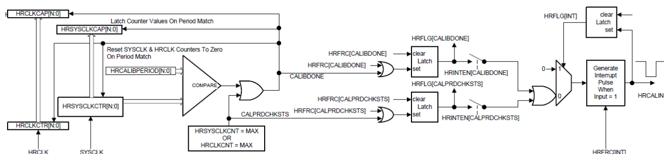
图 6-6. HRCAP 校准
