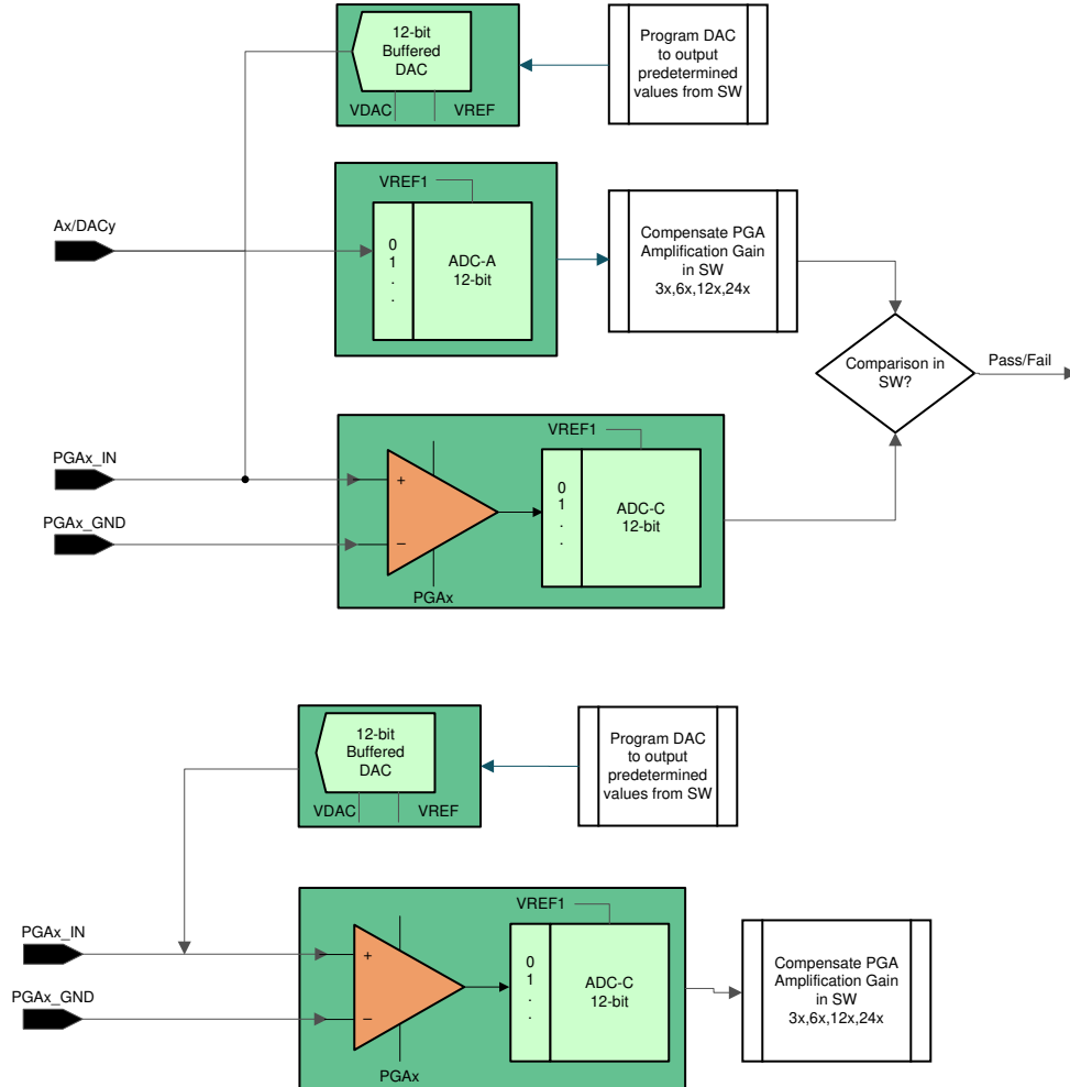
图 6-9. 使用 ADC 和 DAC 来测试 PGA
