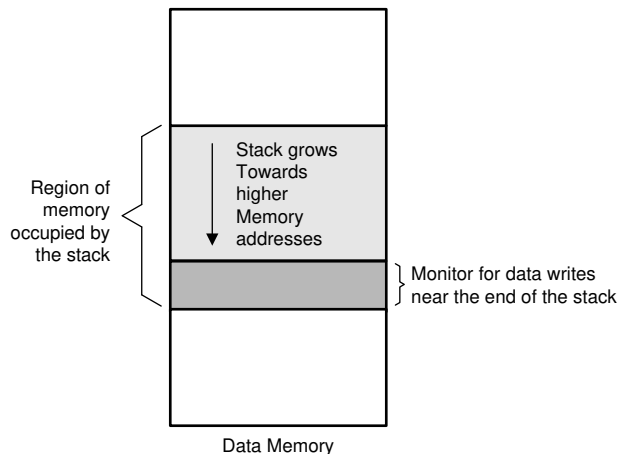
图 6-2. 栈溢出监测
