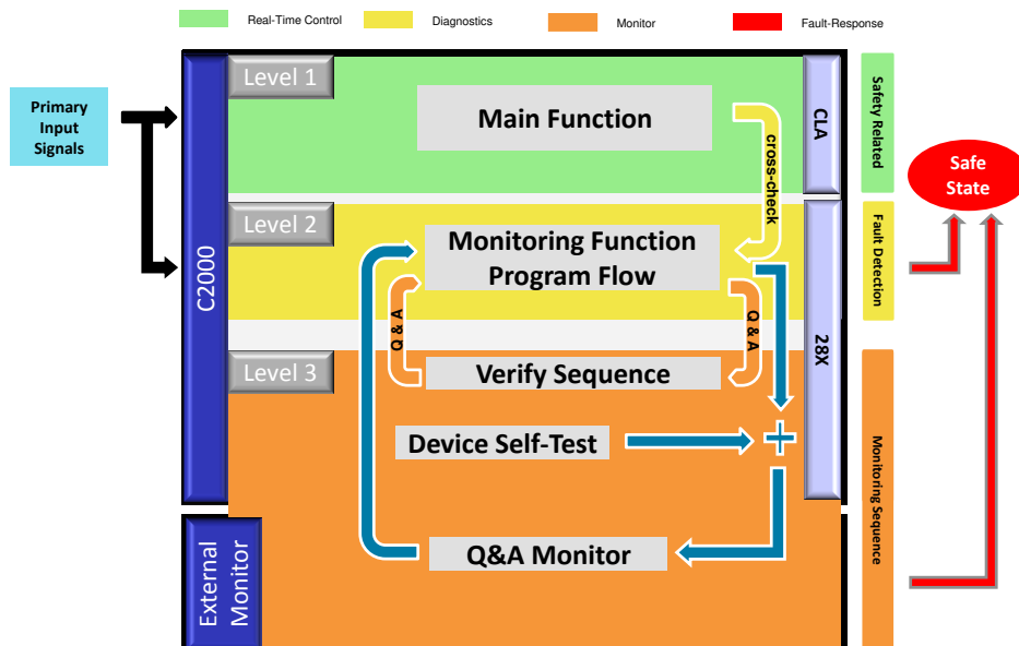
图 4-4. 应用于 F28004x MCU 的 VDA E-Gas 监测概念
