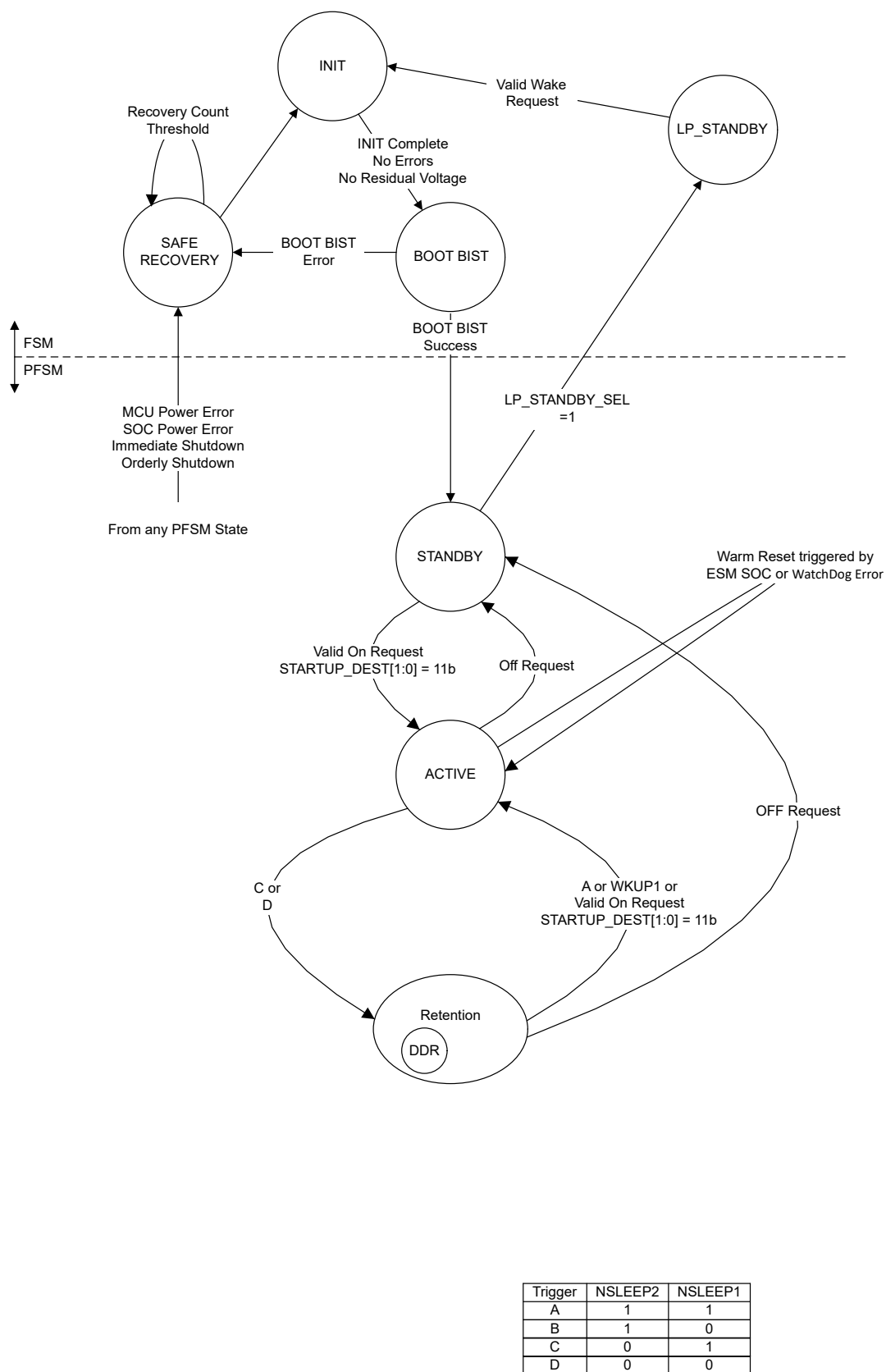
图 6-1. 可预配置有限状态机 (PFSM) 的任务状态和转换
