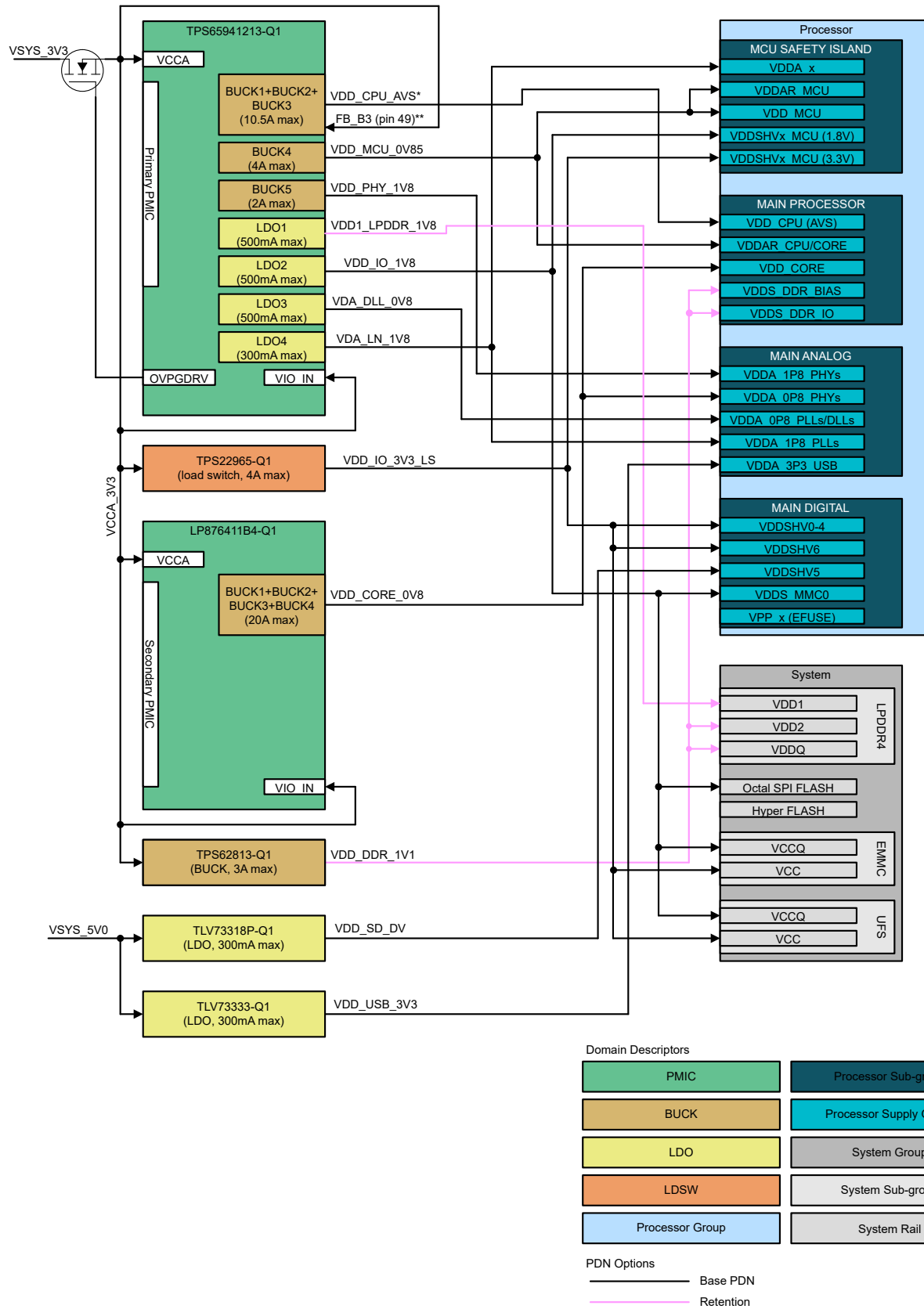
图 3-1. 电源连接
