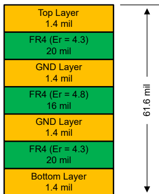
图 4-3. PCB 层堆叠
