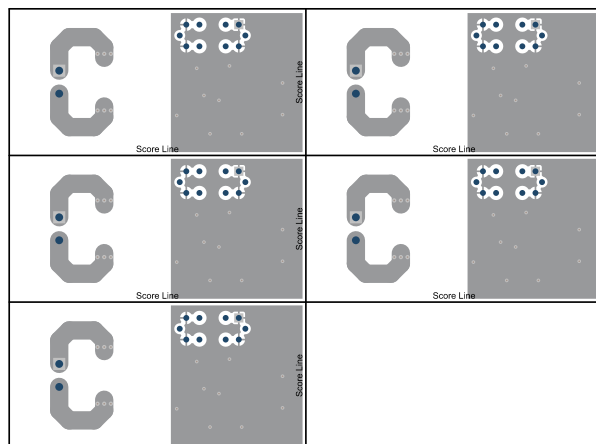
图 5-6. SENS095 底层
