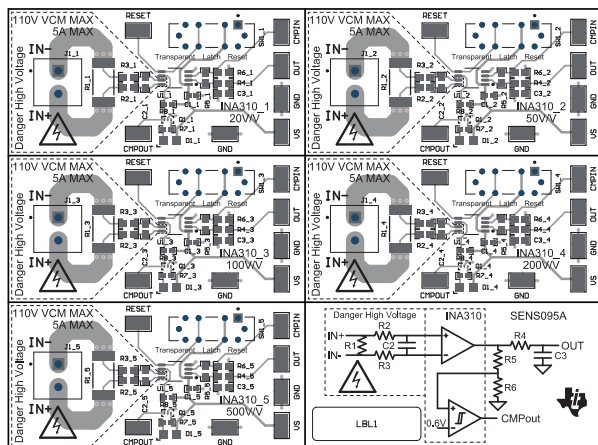
图 5-3. SENS095 顶视图
