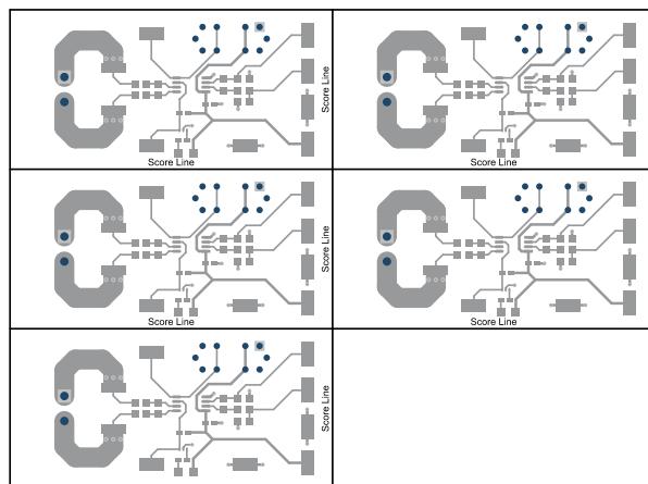
图 5-4. SENS095 顶层
