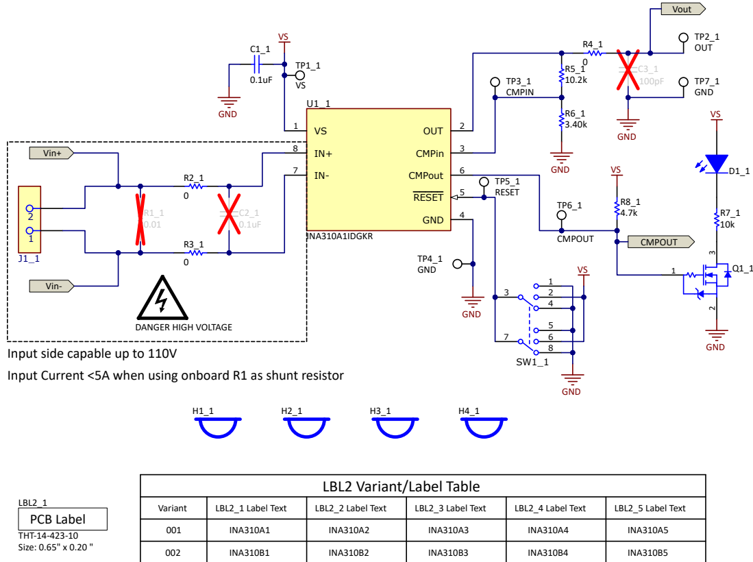
图 5-1. INA310 原理图
